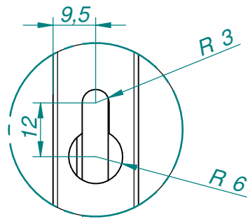
SZCZEGÓŁ B
